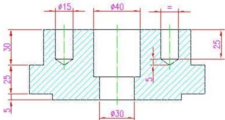
Corte A-a
