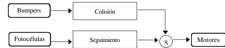
Figura 3. Ejemplo de control reactivo basado en comportamientos
